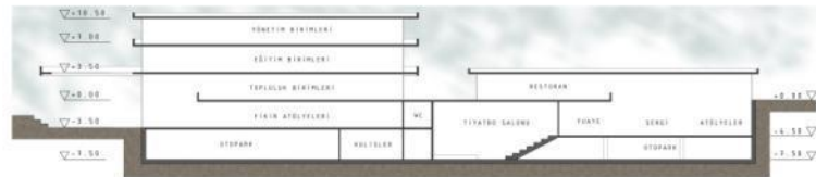
C-C KESİTİ 0:1/200
