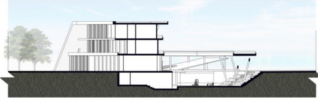
3-3 KESİTİ ÖLÇEK : 1 / 200
