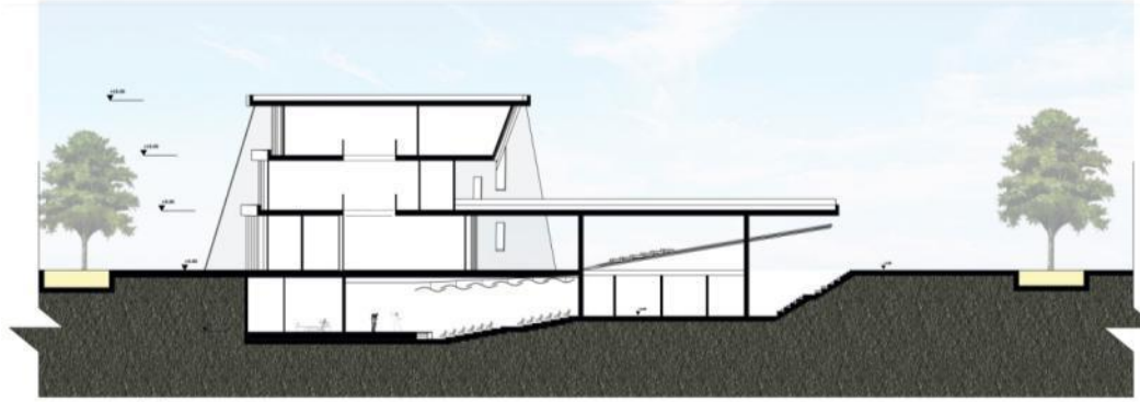
2-2 KESİTİ ÖLÇEK : 1 / 200
