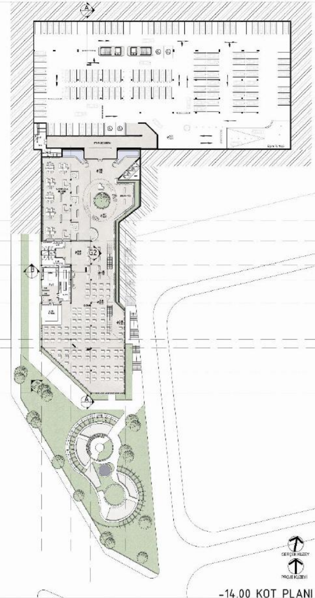
-14.00 KOT PLANI ÖLÇEK:1/200
