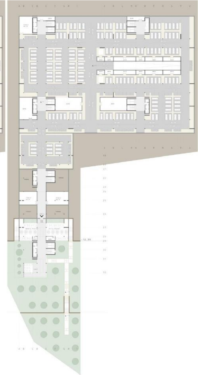
-16.00 KOT PLANI
