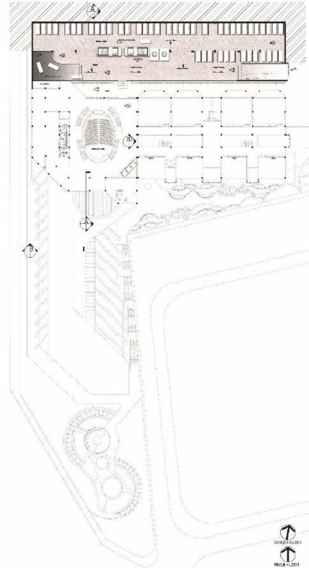
-2.50 & -7.50 KOT PLANI ÖLÇEK:1/200
