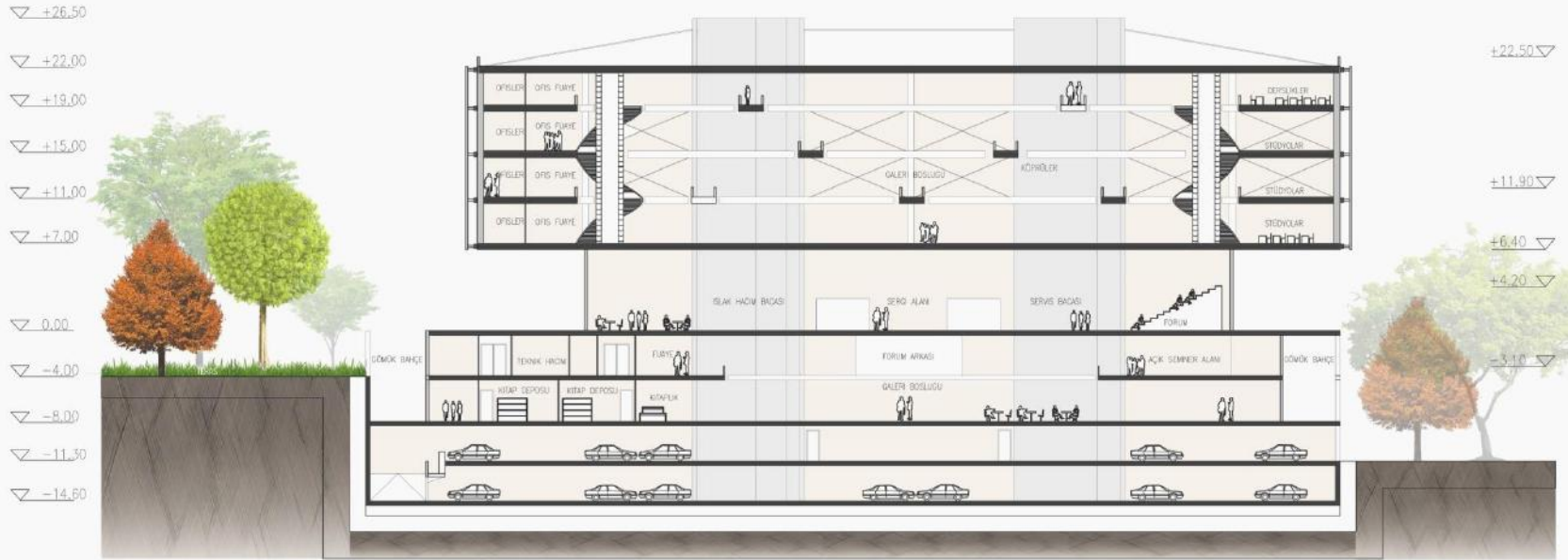
A-A KESİTİ Ö: 1/200
