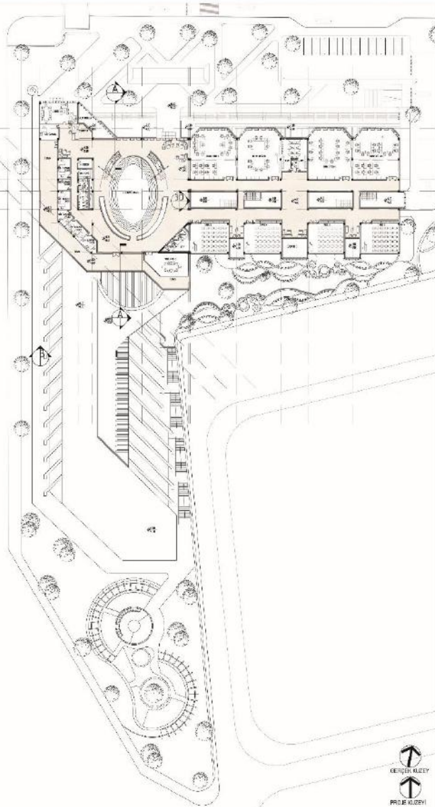
+4.40 KOT PLANI ÖLÇEK:1/200
