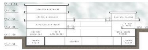
D-D KESİTİ 0:1/200
