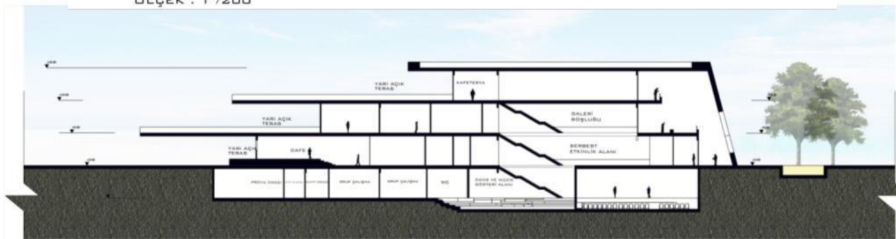
1-1 KESİTİ ÖLÇEK : 1 / 200
