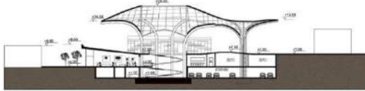
B-B KESİTİ ÖLÇEK: 1/200
