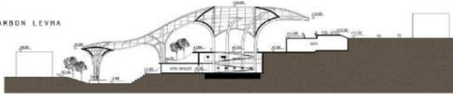
A-A KESİTİ ÖLÇEK: 1/200
