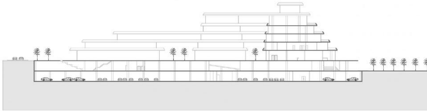
A-A KESİT 1/200
