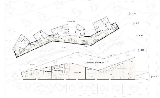
-1.00 KOT PLANI 1/200
