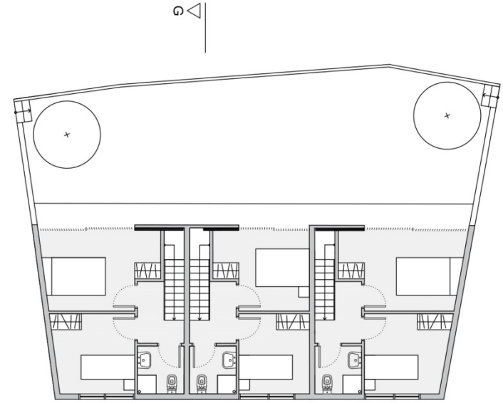
1/100 AİLE KONUTU ZEMİN KAT PLANI
