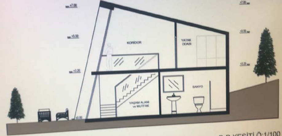
B-B KESİTİ Ö:1/100
