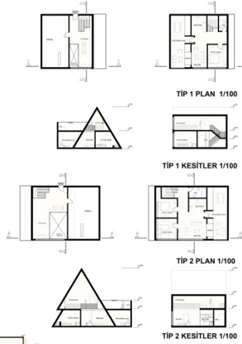
TİP 2 KESİTLER 1/100
