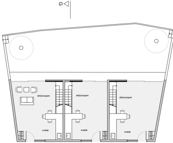
1/100 AİLE KONUTU ZEMİN KAT PLANI
