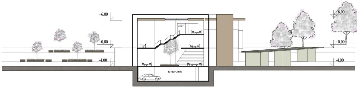
B-B KESİTİ 1/200
