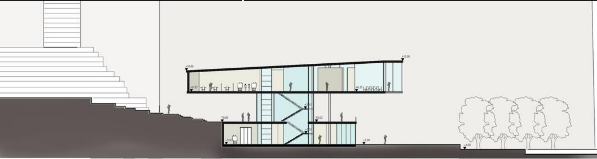
A-A KESİTİ 1/200
