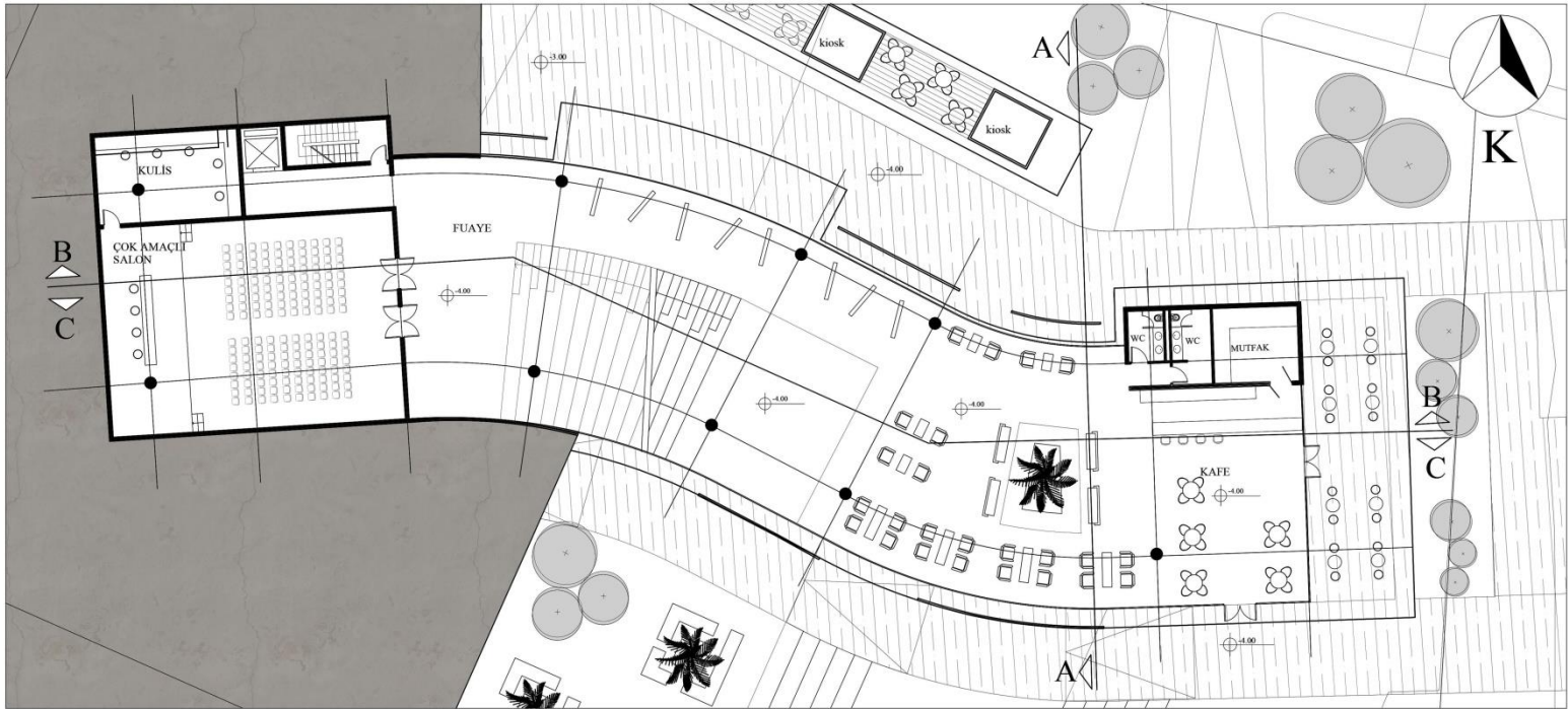
-4.00 KOT PLANI 1/200
