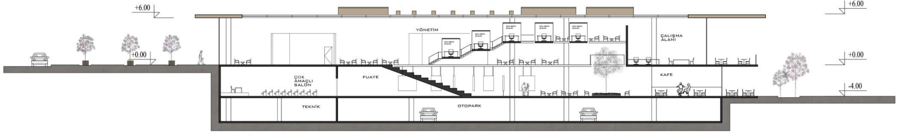
A-A KESİTİ 1/200
