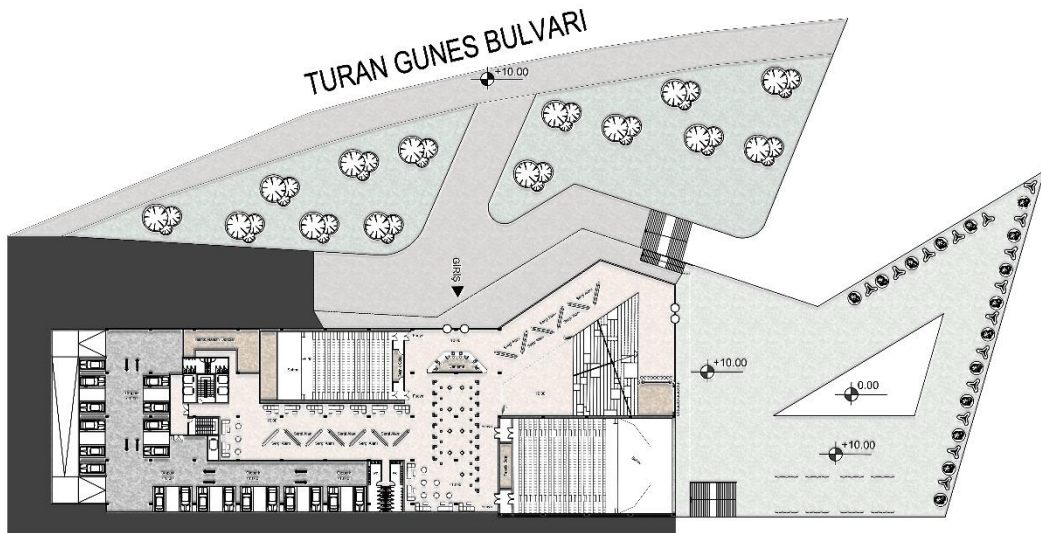
1/200 +10.00 Kotu Planı
