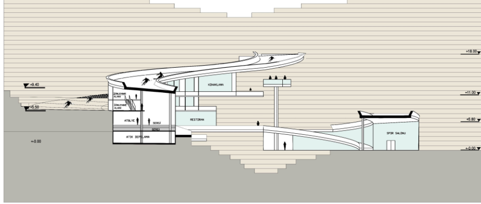
1/200 A-A KESİT
