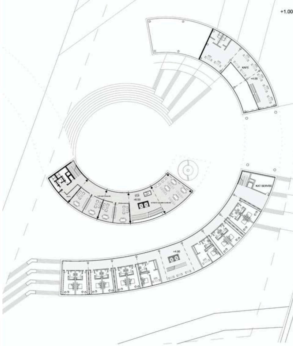
+6.00 KOT PLANI
