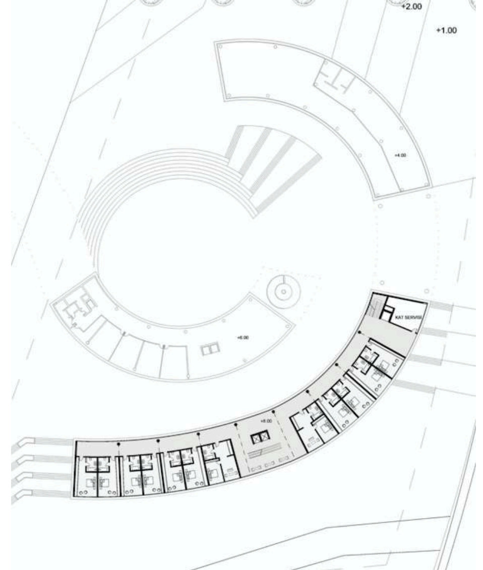
+8.00 KOT PLANI
