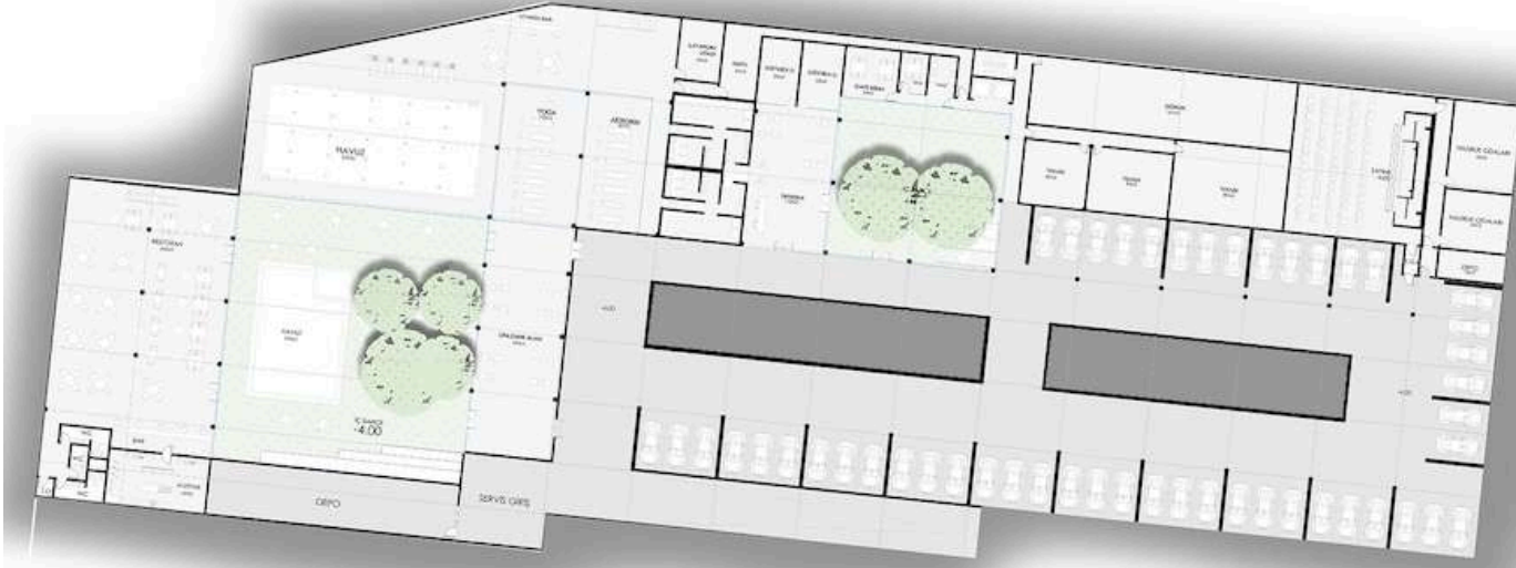
-4.00 KOTU PLANI 1/200
