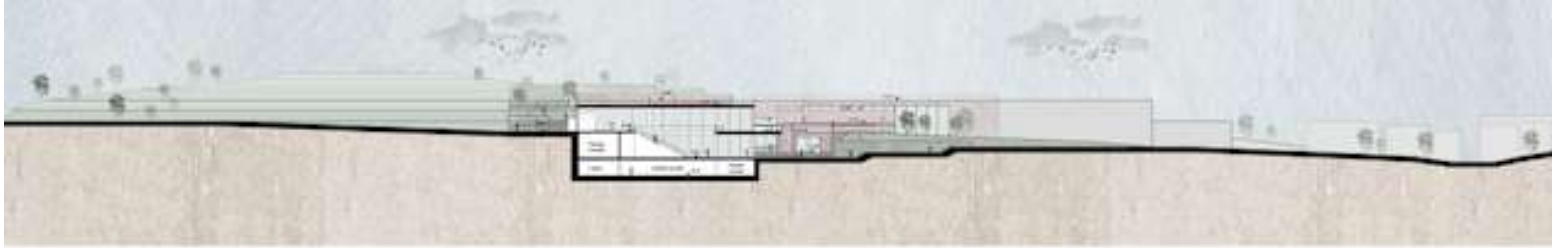
C-C KESİTİ ÖLÇEK: 1/200
