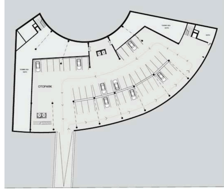
-8.00 KOT PLANI
