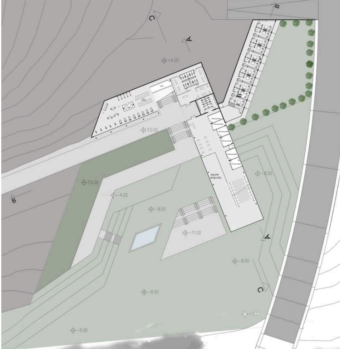
0.00 KOT PLANI ÖLÇEK 1/200
